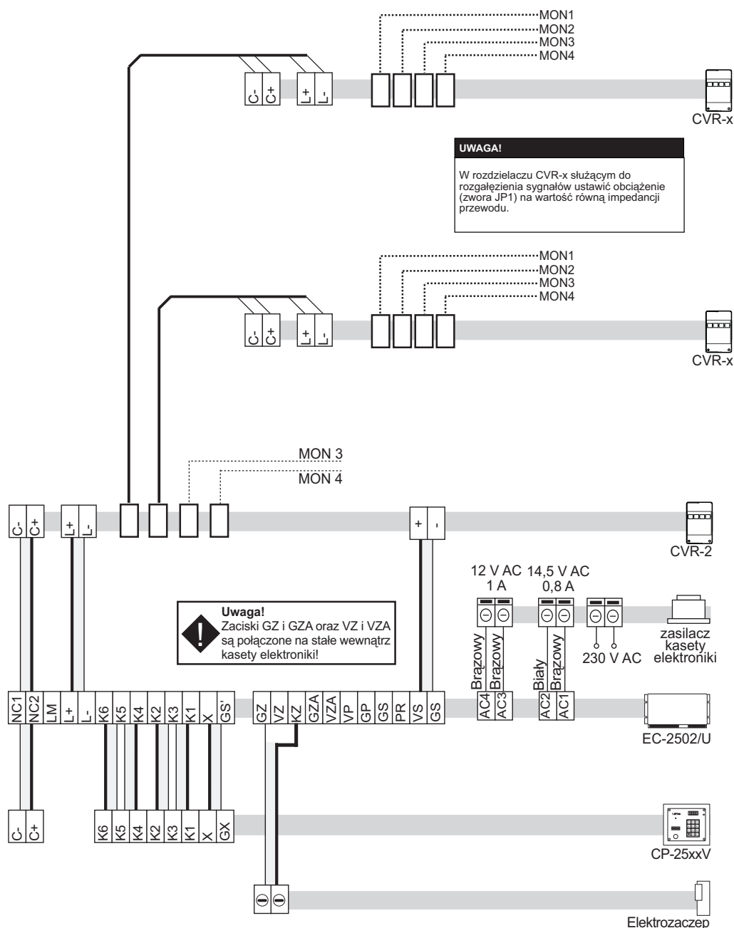
Rysunek 44: Domofon CD-2502 video - rozgałęzienie sygnału przy pomocy rozdzielacza CVR-2
