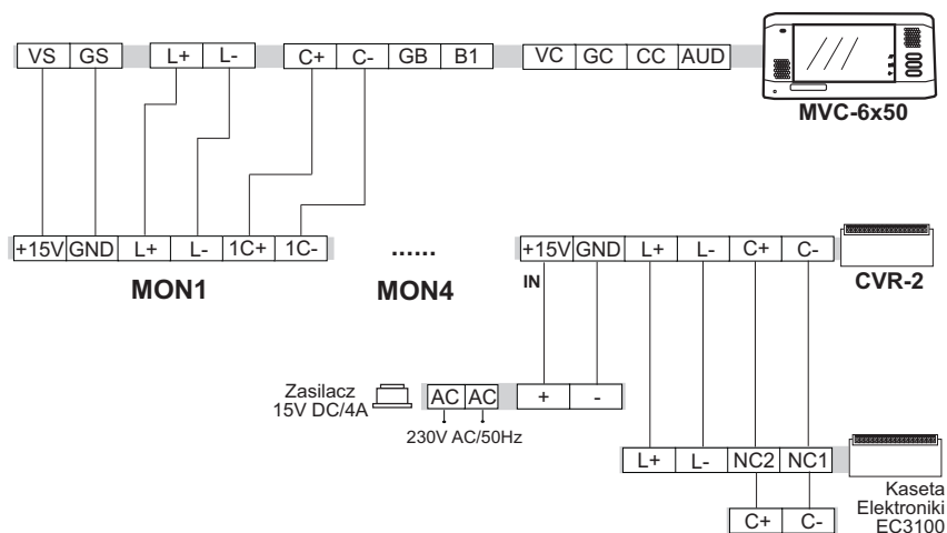
Rysunek 40: System CD-2502 wideo. Podłączenie monitorów poprzez rozdzielacz CVR-2 - zasilanie centralne monitorów.
