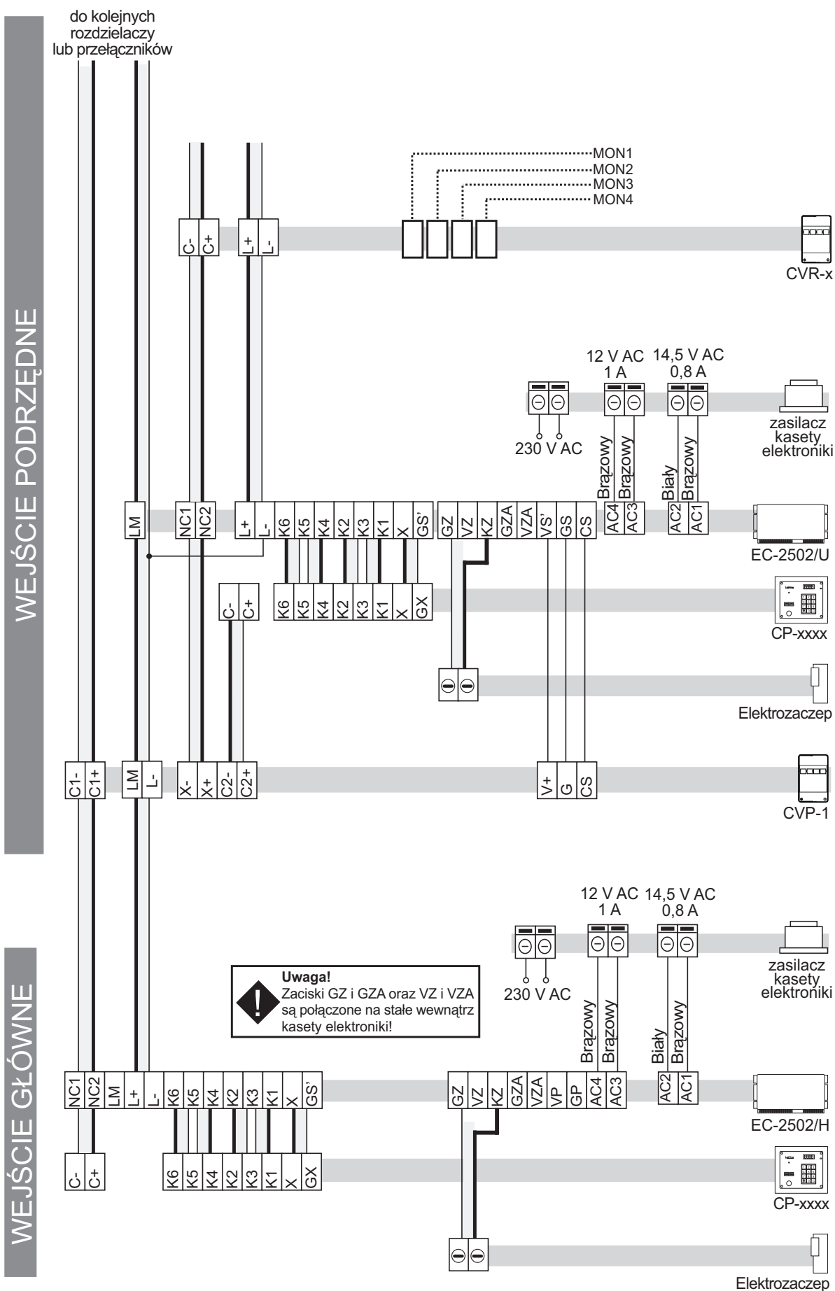
Rysunek 43: Domofon CD-2502 video - system wielowejściowy
