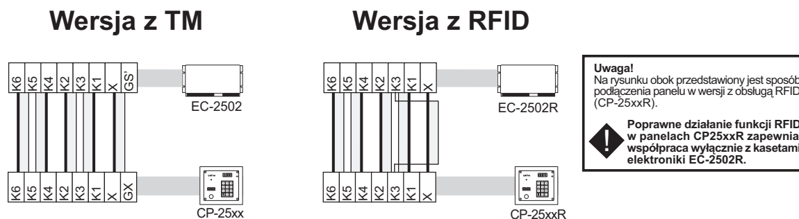
Rysunek 45: Sposób podłączenia kasety elektroniki EC-2502 z panelem CP-2502 w zależności od rodzaju zamontowanego czytnika kluczy elektronicznych.
