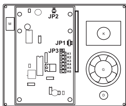
Rysunek 9: Panel zewnętrzny - ustawienie rodzaju zastosowanego wyświetlacza oraz zasilania kamery (tylko w wersji wideo) na przykładzie CP-2502
