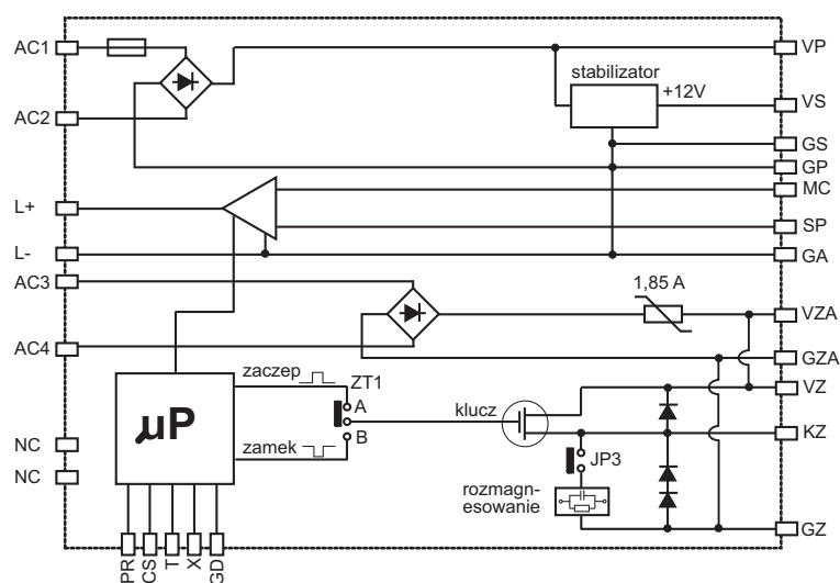
Rysunek 38: Schemat blokowy kasety elektroniki
